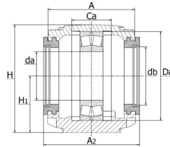
Labyrint afdichting
