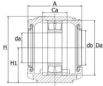
Vilt-, rubber-, V-ring afdichting
