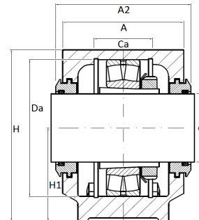
Labyrint afdichting
