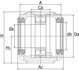
Labyrint afdichting
