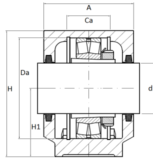
Vilt-, rubber-, V-ring afdichting
