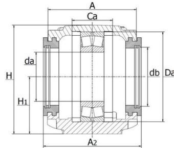
Labyrint afdichting
