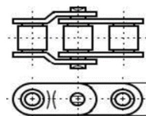
Dubbele verloopschakel
