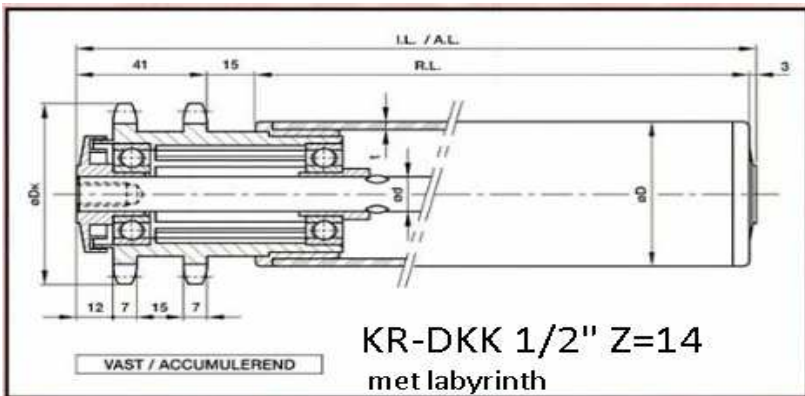
DKK 1/2" Z=14 dub labyrinth (art 78000101) Kunststof rol Ø50x2,8 vv kunststof DKK ketting wiel met stofkap labyrinth
