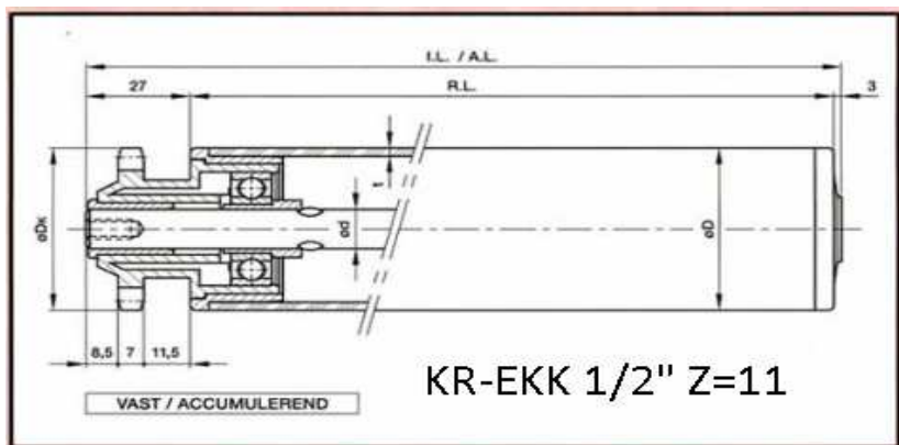
EKK 1/2" Z=11 enkel (art 78000100)
