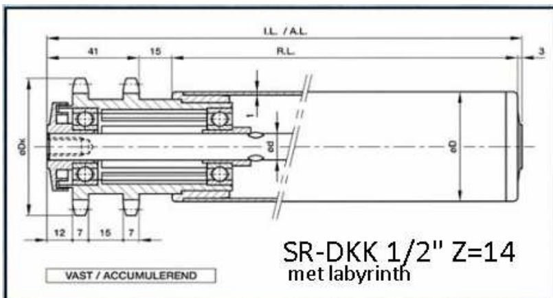
DKK 1/2" Z=14 dub labyrinth (art 78000101)
