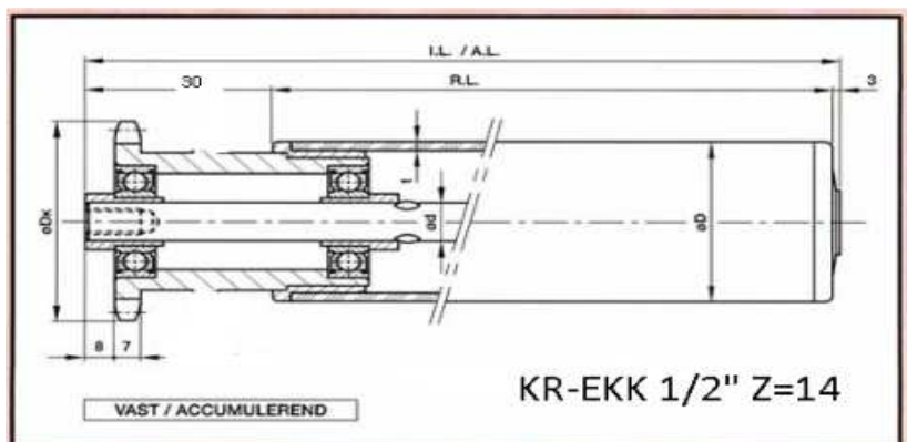
EKK 1/2" Z=14 enkel (art 78000105)
