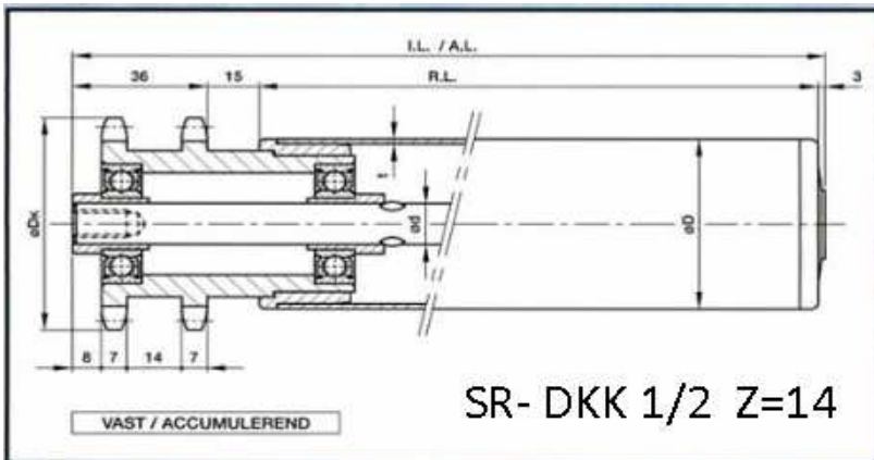
DKK 1/2" Z=14 dubbel (art 78000103)
