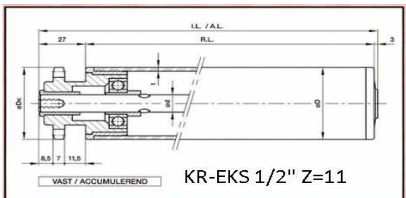
EKS 1/2" Z=11 enkel (art 78000107)
