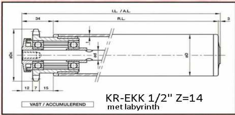
EKK 1/2" Z=14 enk labyrinth (art 78000102) Kunststof rol Ø50x2,8 vv kunststof EKK ketting wiel met stofkap labyrinth
