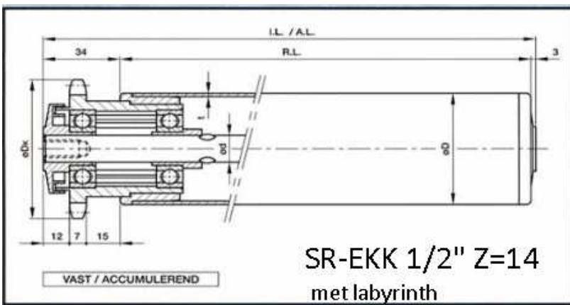
EKK 1/2" Z=14 enk labyrinth (art 78000102)
