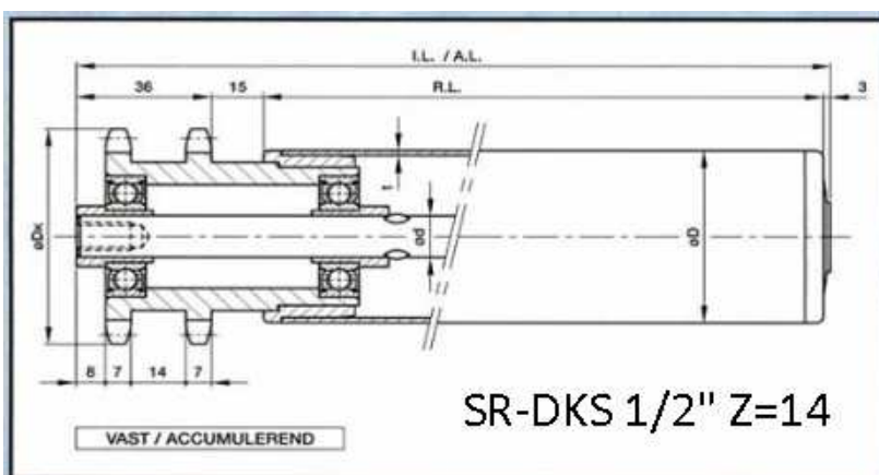
DKS 1/2" Z=14 dubbel (art 78000109)
