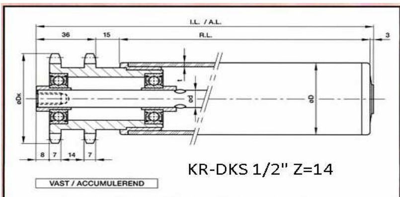
DKS 1/2" Z=14 dubbel (art 78000109) Kunststof rol Ø50x2,8 vv stalen DKS ketting wiel
