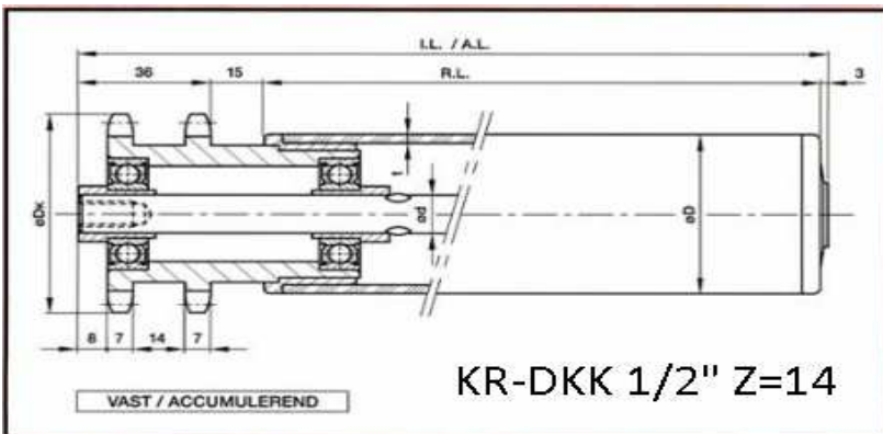
DKK 1/2" Z=14 dubbel (art 78000103) Kunststof rol Ø50x2,8 vv kunststof DKK ketting wiel
